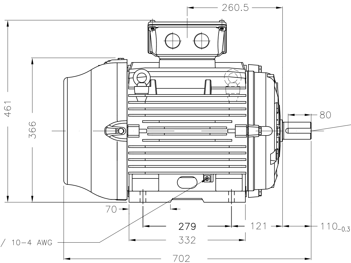
Center hole DM16 WEG TBG12 (DIN 332)
